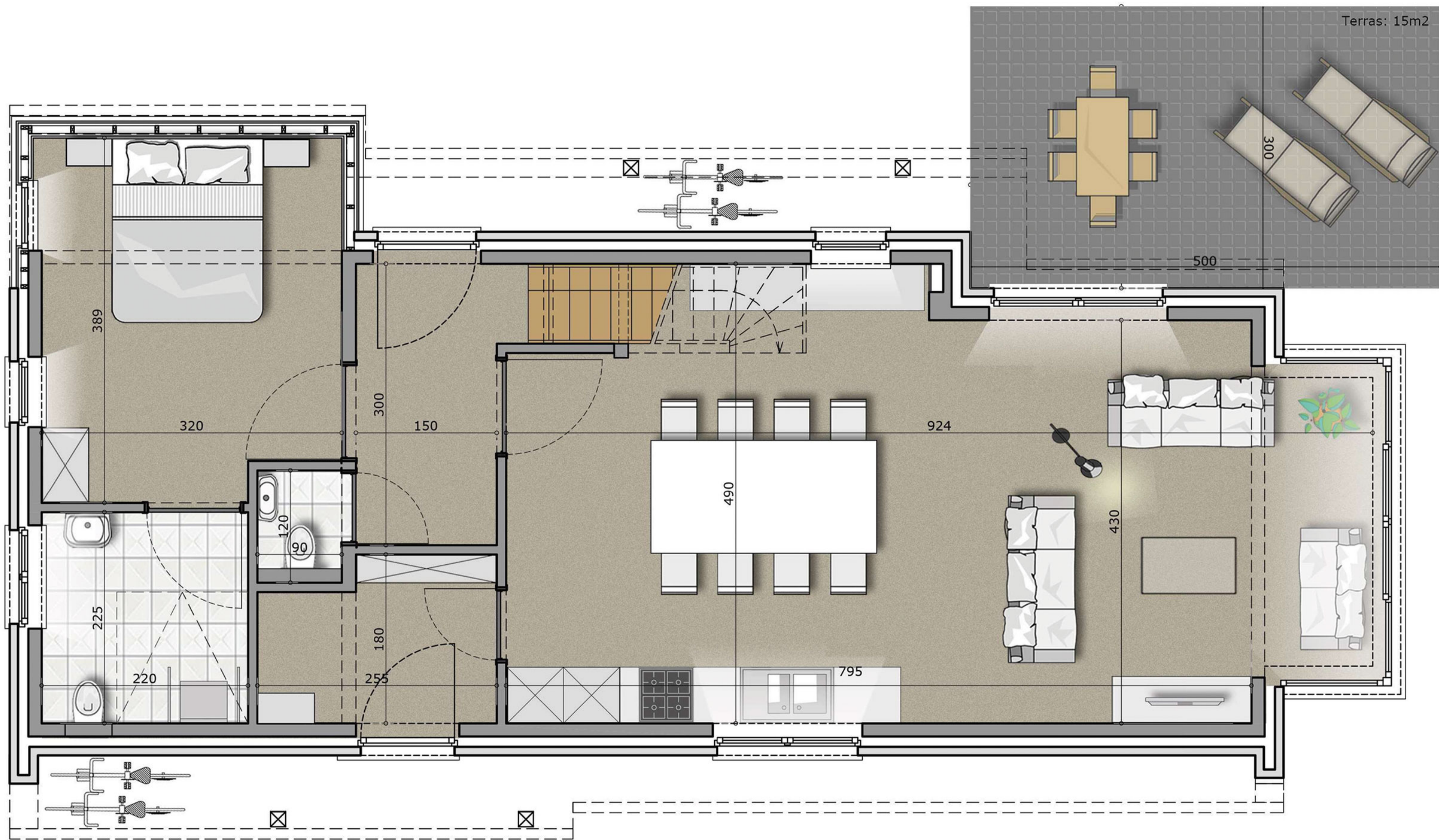
8 PERSOONSWONING gelijkvloerse verdieping (82,64 m 2 ) - schaal 1/50 bruto-oppervlakte woning : 156,37 m 2
